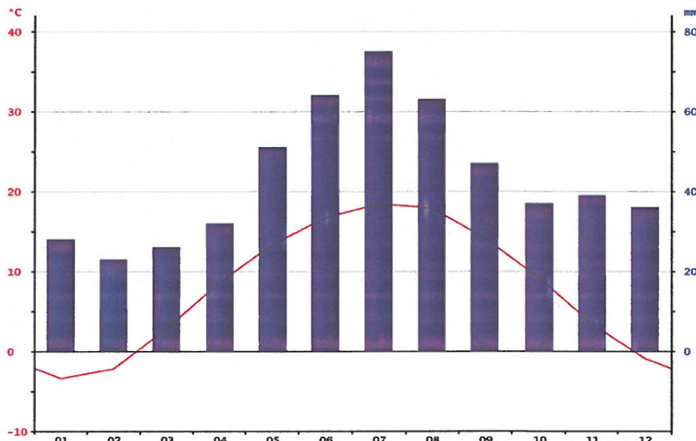
Wykres 2. Wykres klimatyczny dla miejscowości Ostrowite
