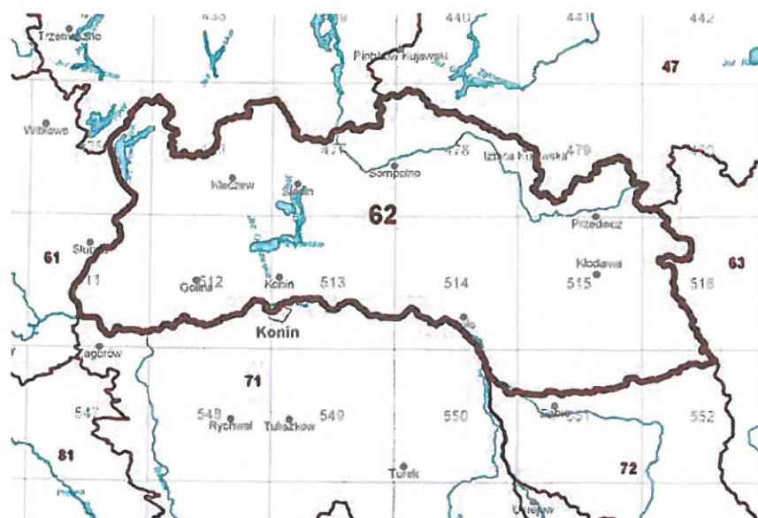
Rysunek 8. Zasięg terytorialny JCWPd nr 62
