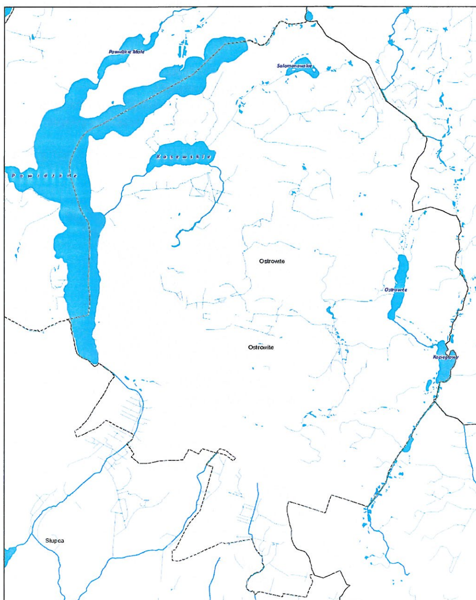
Rysunek 6. Sieć hydrograficzna Gminy Ostrowite
